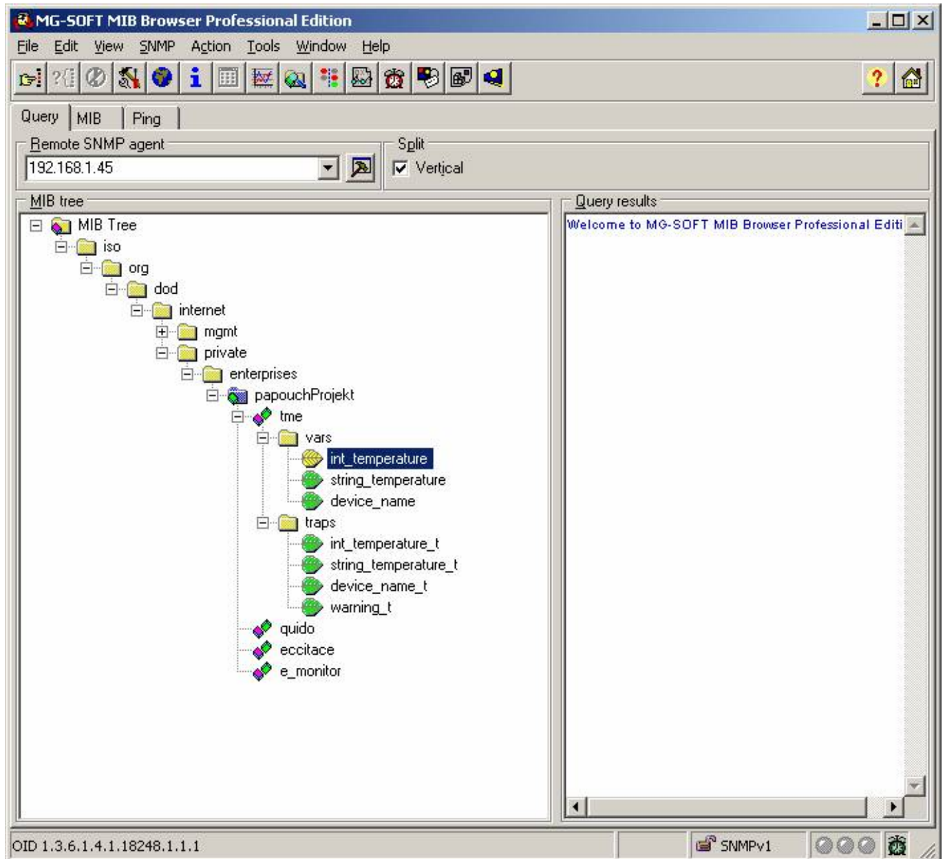
Fig. 37 – MIB tree
